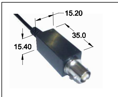
DETALHE DA CAIXA COM CONECTOR BNC
